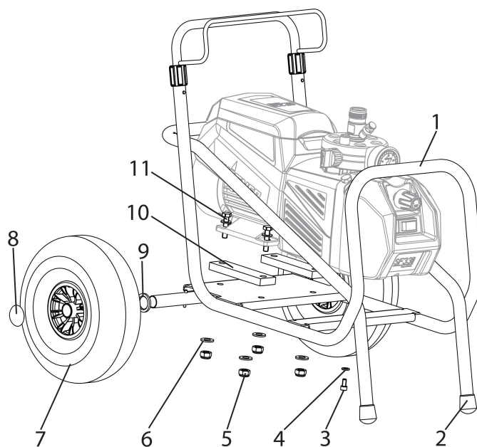
Reservebillede, vogn
