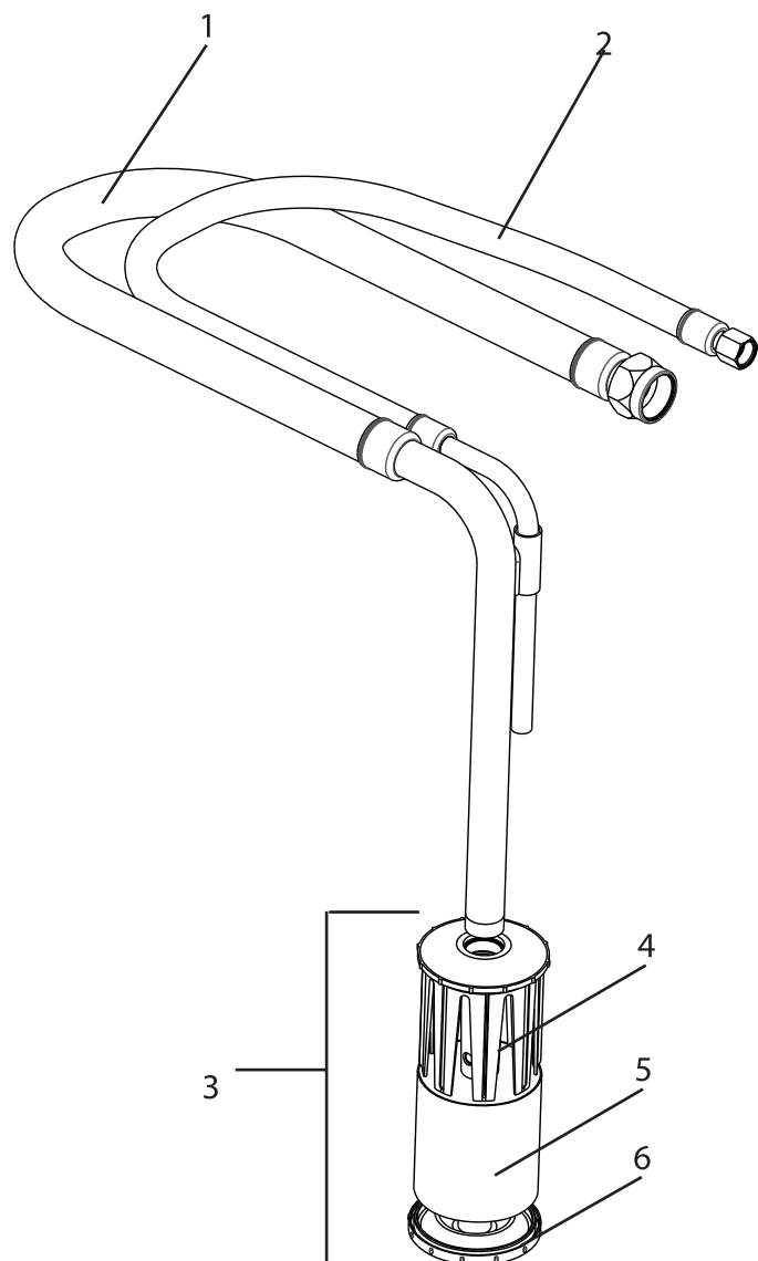
Reservedelsbillede, indsugningssystem
