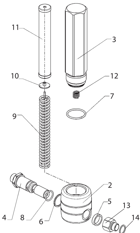
Reservebillede, højtryksfilter
