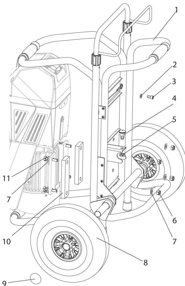
Reservebillede, vogn
